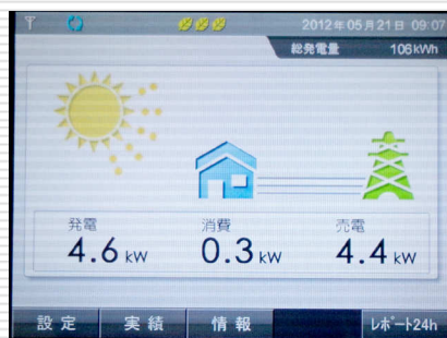
2012.05.17～稼働を開始した 麻布十番本社ビル屋上に設置した 太陽光パネル54枚 9.8kw
